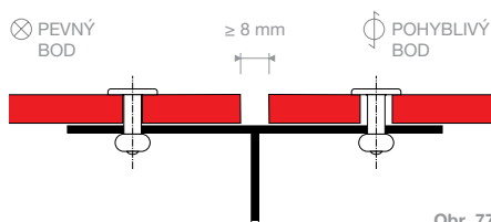
PŘÍKLAD VERTIKÁLNÍ SPÁRY
