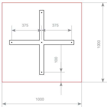
PŘÍKLAD STOLOVÉ DESKY-PŘESAŘ
