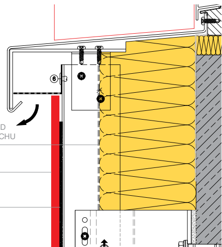
VODOROVNÁ SPÁRA A102
