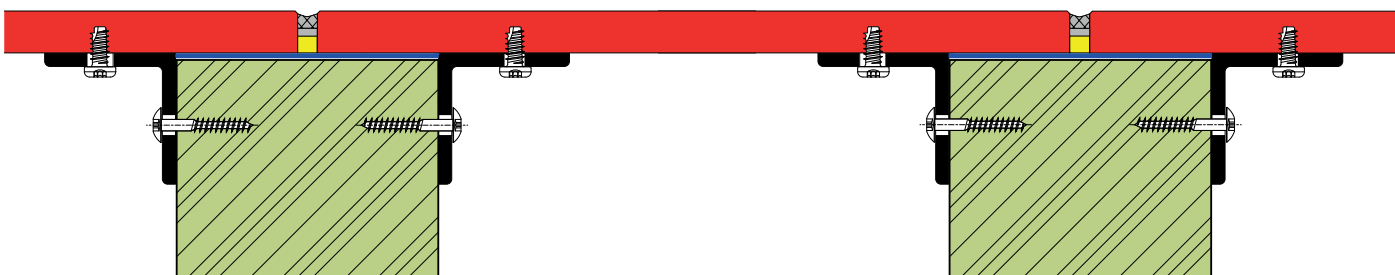
BALKONOVÁ PODLAHOVÁ DESKA UPEVNĚNÁ NA DŘEVĚNÉM TRÁMU (NEPŘIZNANÉ UPEVNĚNÍ – ŠROUBEM)
